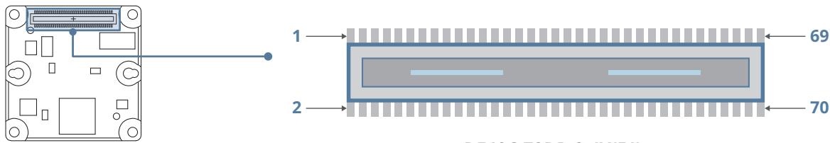
DF40C-70DP-0.4V(51)
